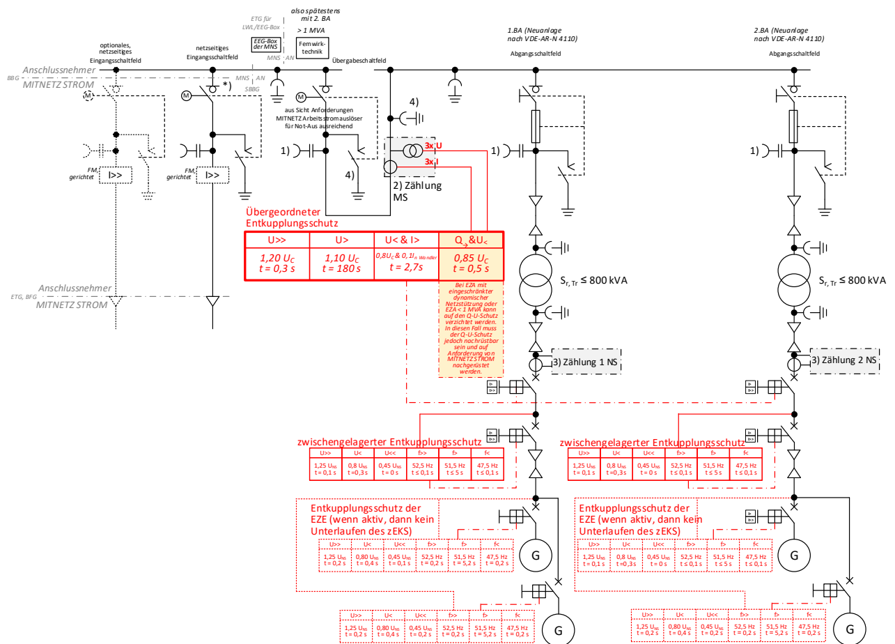
Abb. 32: (ehemals D4e): \leq 20 -kV-Anbindung von zwei Bauabschnitten einer PV-Anlage mit je 750 kVA (spätestens ab 2.BA mit FWT, in diesem Fall im 1.BA mit FRE)
