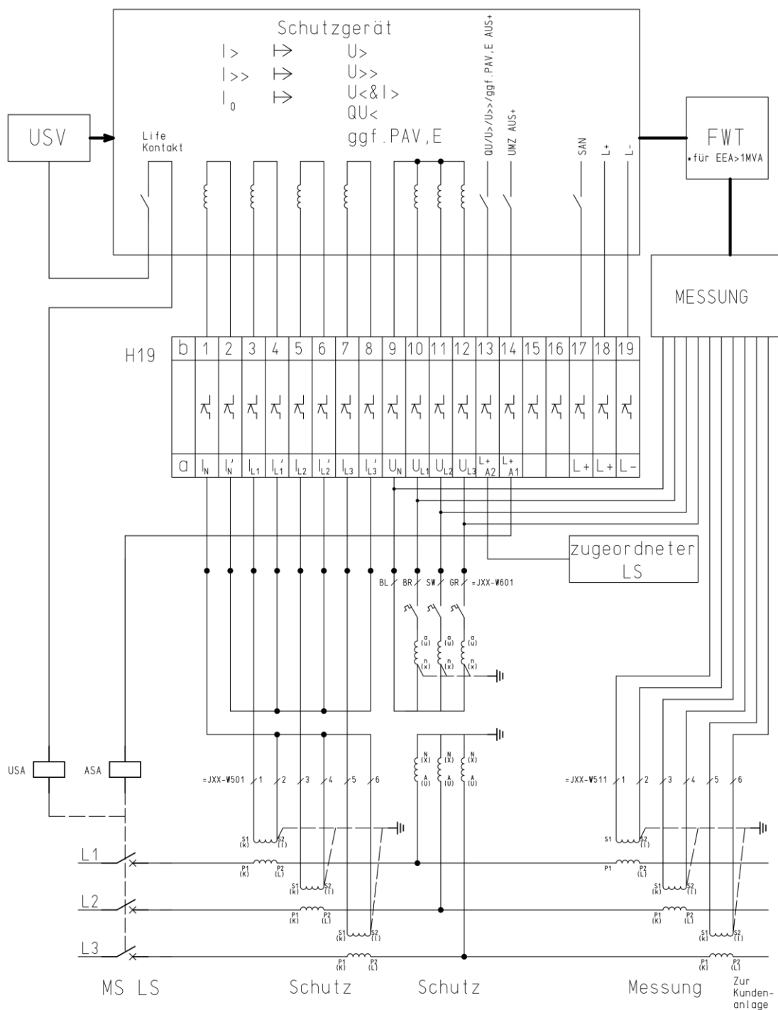
Abb. 46: Wandlerverdrahtung Anbindung UMZ / übergeordneter Entkupplungsschutz
