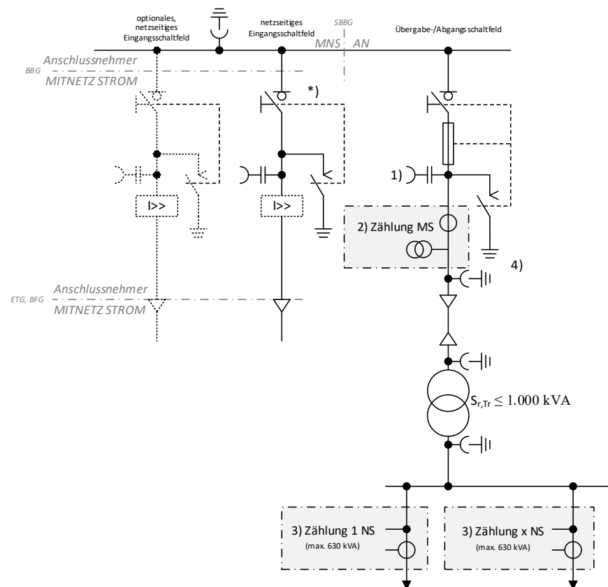
Abb. 23: (ehemals D1a): ≤ 20-kV-Anbindung mit einem Abgangsfeld; Transformator ≤ 1 MVA (z.B. 630 kVA)
